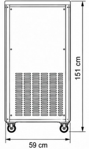
ARKA GÖRÜNÜŞ
