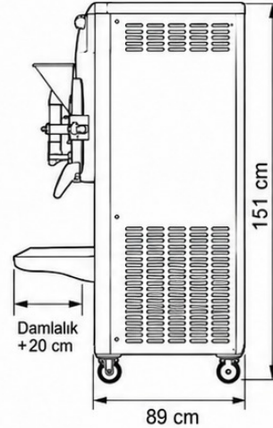
YAN GÖRÜNÜŞ
