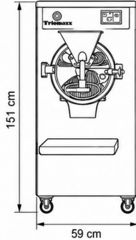
ÖN GÖRÜNÜŞ
