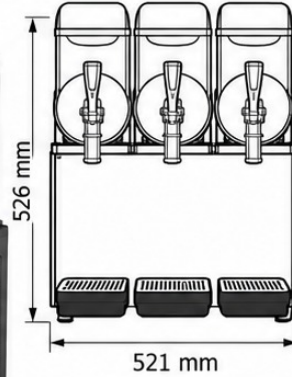
ÖN GÖRÜNÜŞ
