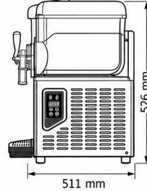
YAN GÖRÜNÜŞ
