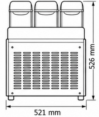
ARKA GÖRÜNÜŞ
