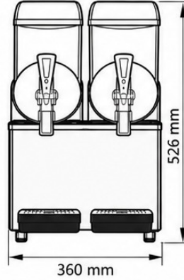
ÖN GÖRÜNÜŞ
