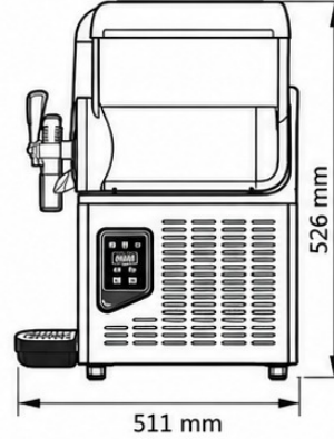
YAN GÖRÜNÜŞ
