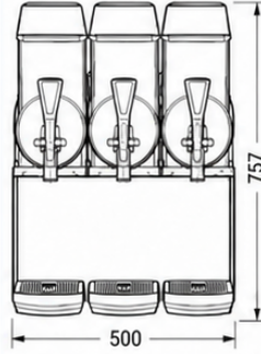
ÖN GÖRÜNÜŞ
