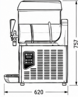
YAN GÖRÜNÜŞ
