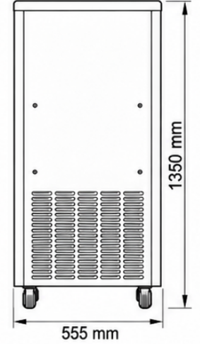
ARKA GÖRÜNÜŞ
