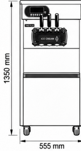
ÖN GÖRÜNÜŞ
