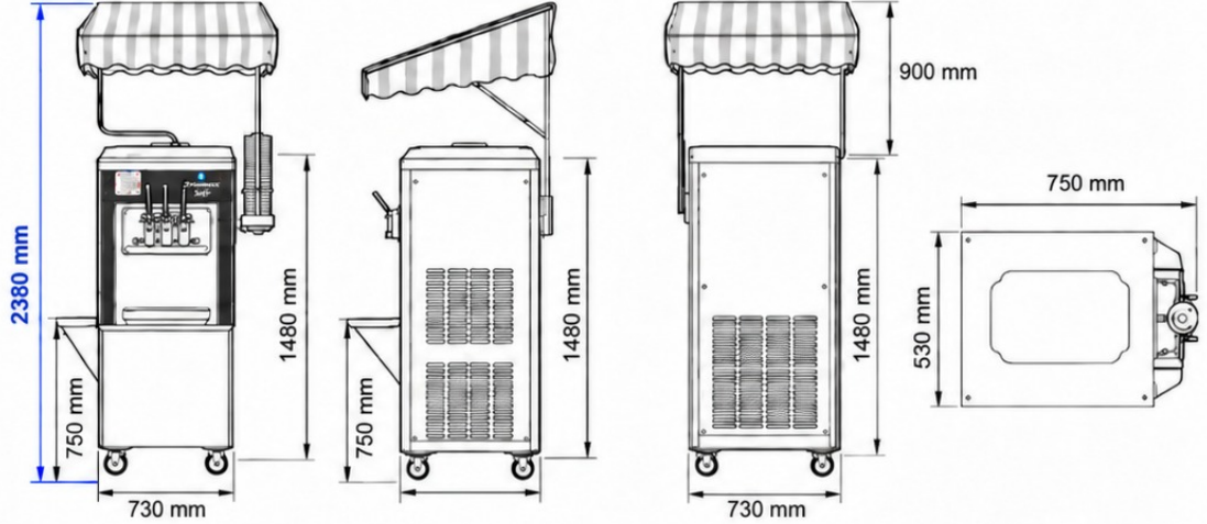
ÖN GÖRÜNÜŞ
